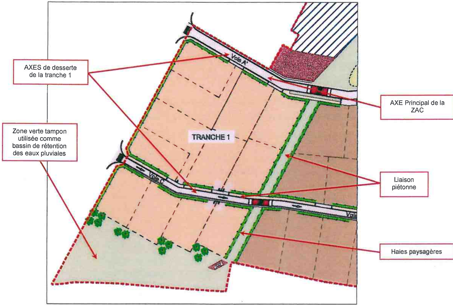
Extrait de plan : tranche1
